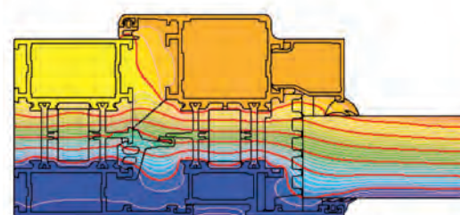
przykładowy rozkład izoterm dla złożenia ościeżnicy i skrzydła okiennego systemu IP i+ (IP 011 + IP 021)
